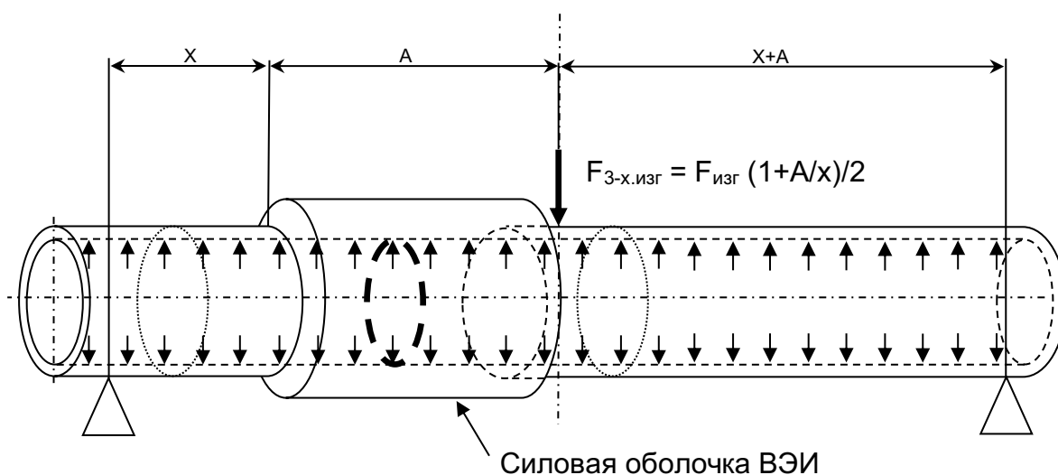
Рисунок 2 – Схема испытания при трехточечном изгибе
