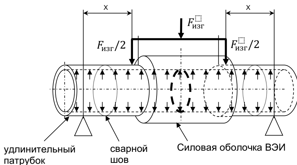
Рисунок 1 – Схема испытания при четырехточечном изгибе
